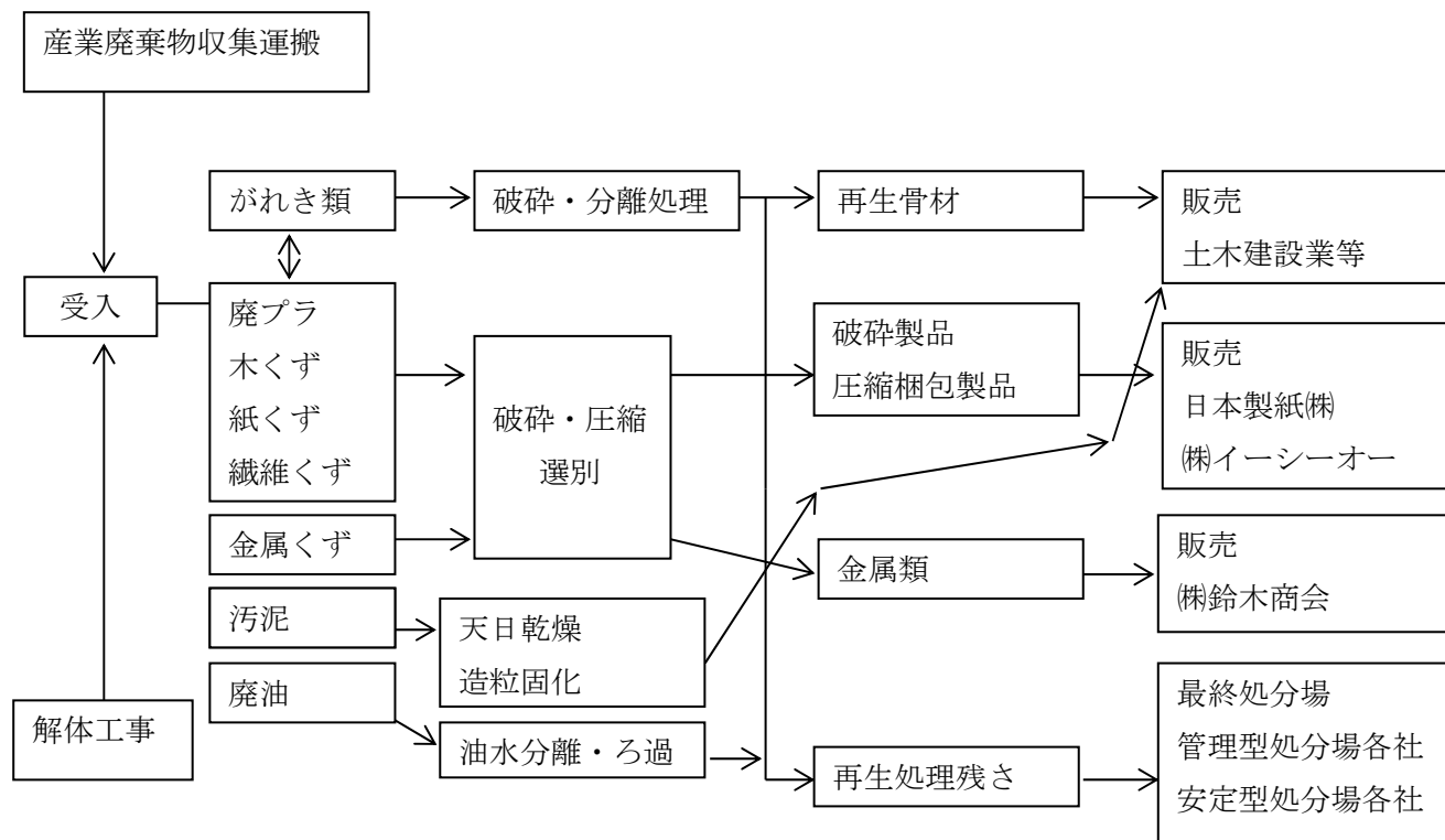
産業廃棄物処理工程図
